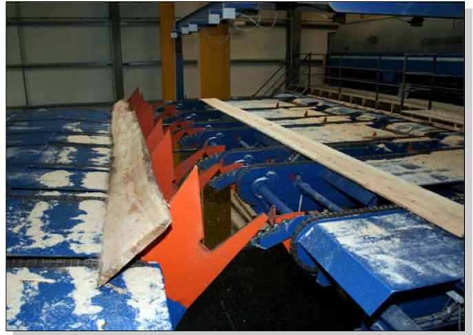
Brettwender einer im sitzen zu bedienenden Besäumanlage
